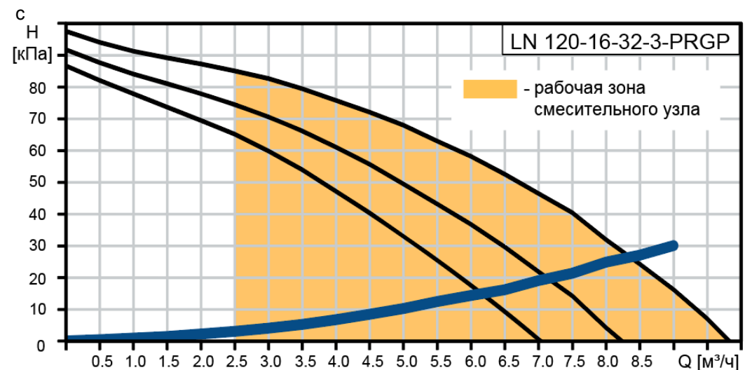
График рабочих характеристик:
