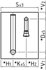
Вид со стороны коллектора
