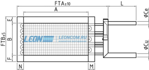
Вид со стороны коллектора
